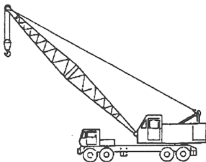
Sobre ruedas, desplazamiento rápido, de estructura giratoria y pluma telescópica.
